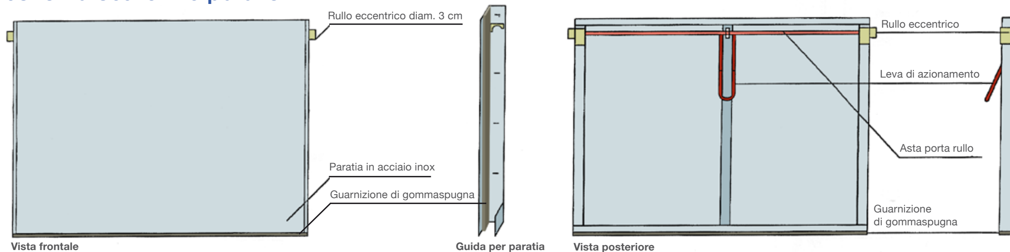
2) Portare la paratia in posizione verticale ancorando i rulli alla guida fissa.
